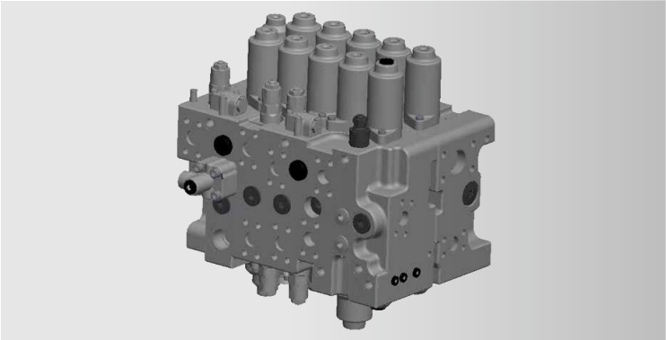
三一主阀采用于川崎制定开发产品，新增加了中位油路截断、斗杆2阀芯电控等功能，更适用于中国工况，压力损失小，能耗低。
